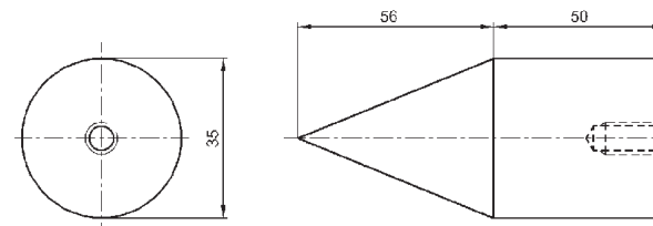
Particolari della sonda di prova Dimensioni in mm
