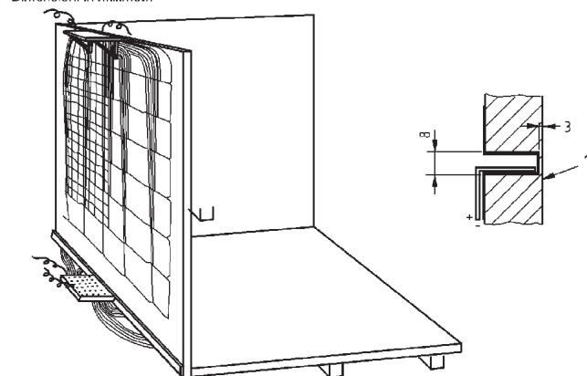
a) disposizione delle termocoppie
