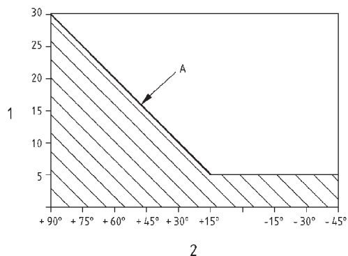
figura C.3 Rapporto tra terminale e direzione del vento per la prova del vento
