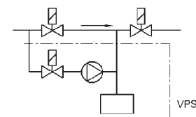
figura 2c Esempio di VPS con valvole parzialmente integrate
