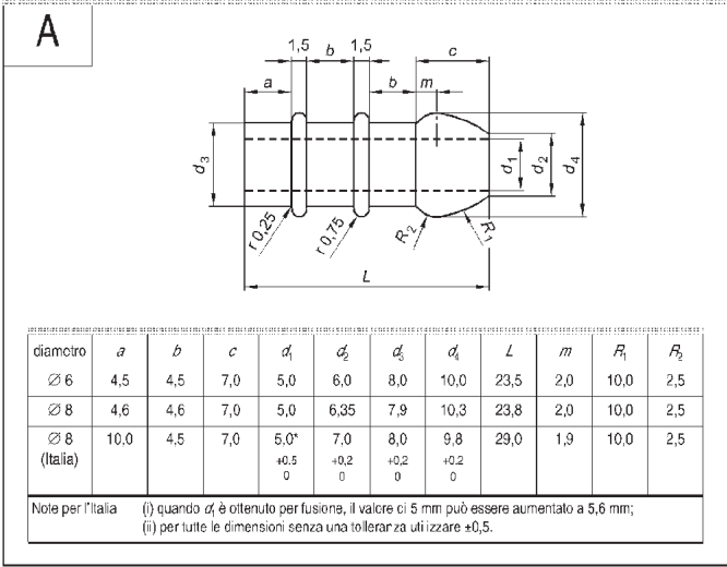
figura B.1 Portagomma
