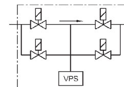
figura 2b Esempio di VPS con valvole integrate
