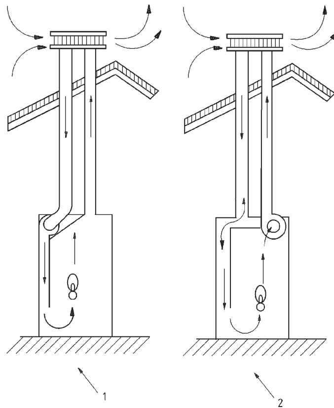
figura B.3 Apparecchi di tipo C 3
