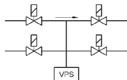
figura 2a Esempio di VPS con valvole esterne da monitorare
