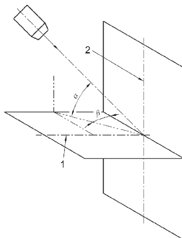
figura 3 Disposizione dell'apparecchiatura di prova per apparecchi di tipo C 1
