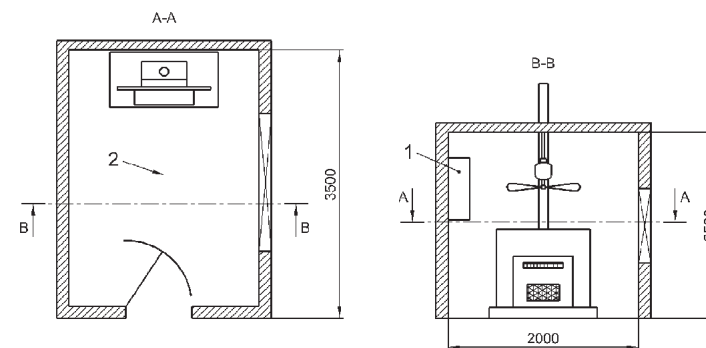
figura 9 Dispositivo di sicurezza per i prodotti della combustione - Apparecchiatura di prova (vedere 7.9.2.3.2)
