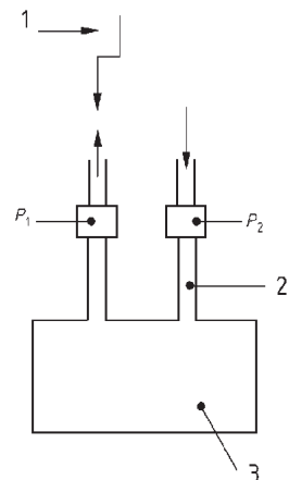
b) posizione dell'orifizio tarato regolabile
