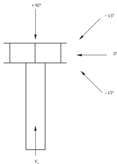
figura C.3 Rapporto tra terminale e direzione del vento per la prova del vento
