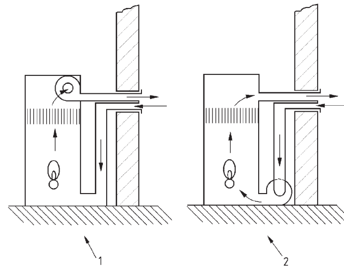
figura B.2 Apparecchi di tipo C 1
