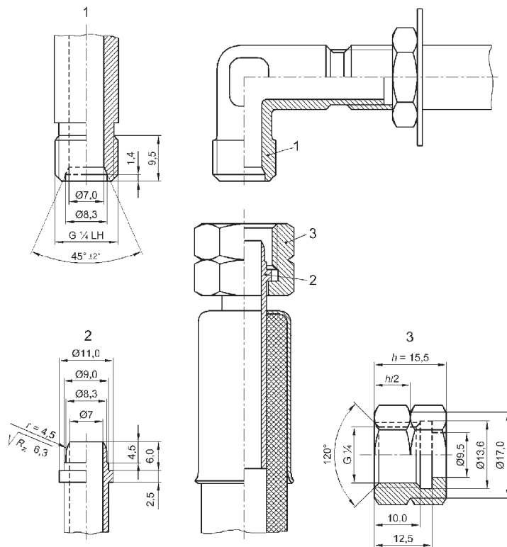
figura A.2 Raccordo Legenda 1 Dettaglio 1 2 Dettaglio 2 3 Dettaglio 3 Dimensioni in mm
