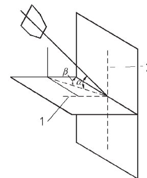
figura 4 Disposizione dell'apparecchiatura di prova per apparecchi di tipo C
